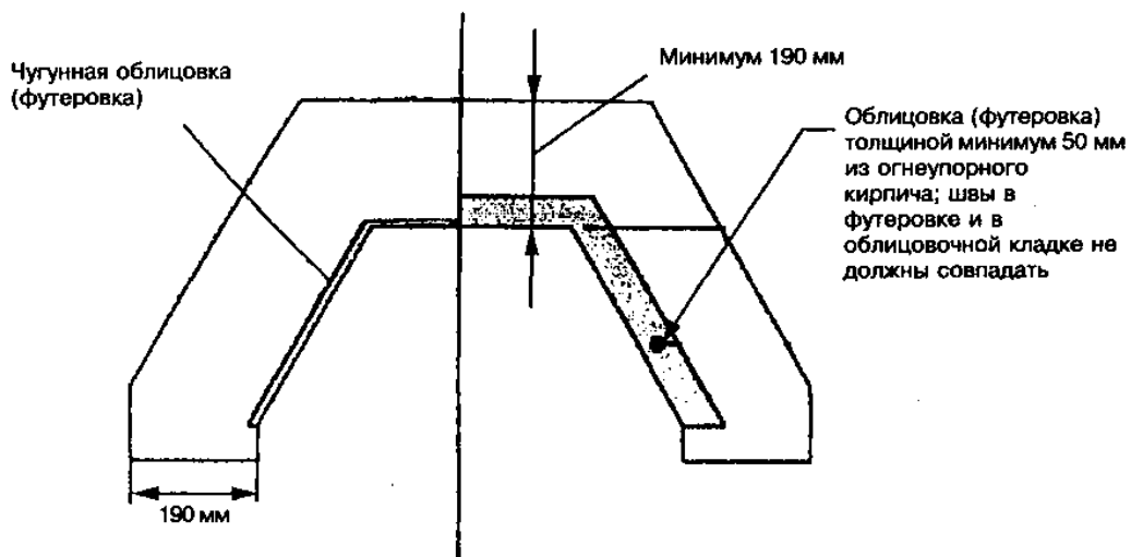
Рисунок 7.5 — Футеровка камина
