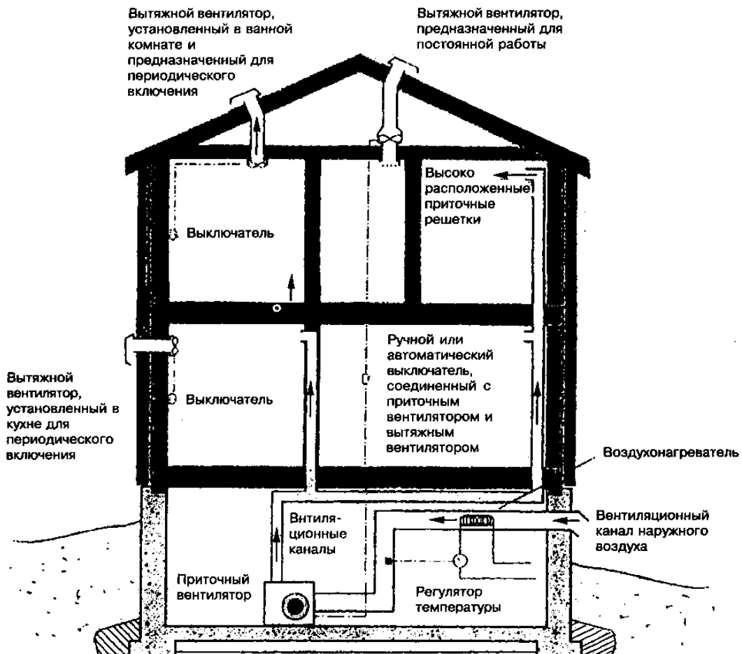
Рисунок 7.2 — Система воздушного отопления с принудительной циркуляцией воздуха,
