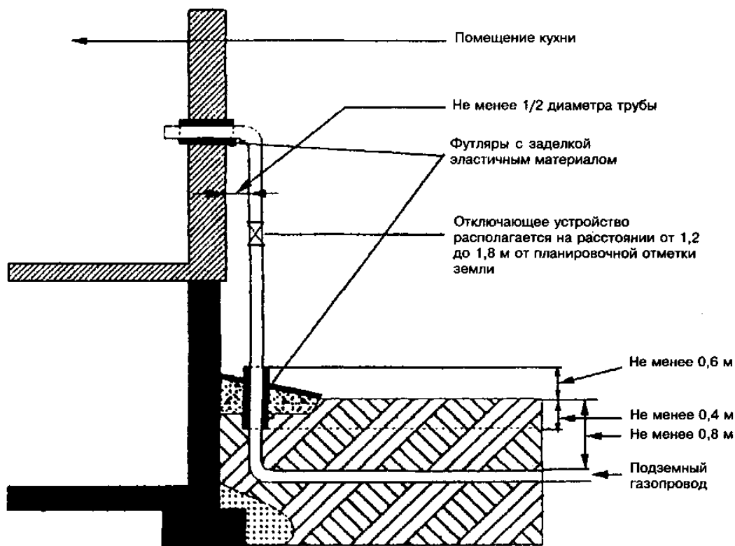
Рисунок 9.1 — Газовый ввод
