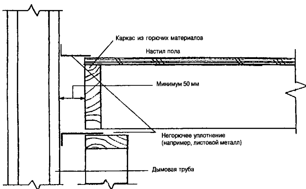
Рисунок 7.8 — Расстояние от дымовой трубы до строительных конструкций
