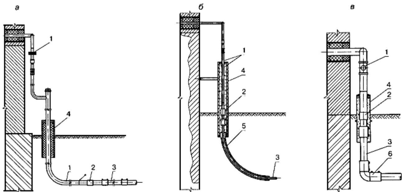
а - стальной цокольный ввод; б - полиэтиленовый ввод, выполненный свободным изгибом трубы; в - полиэтиленовый ввод, выполненный при помощи отвода с 3Н
