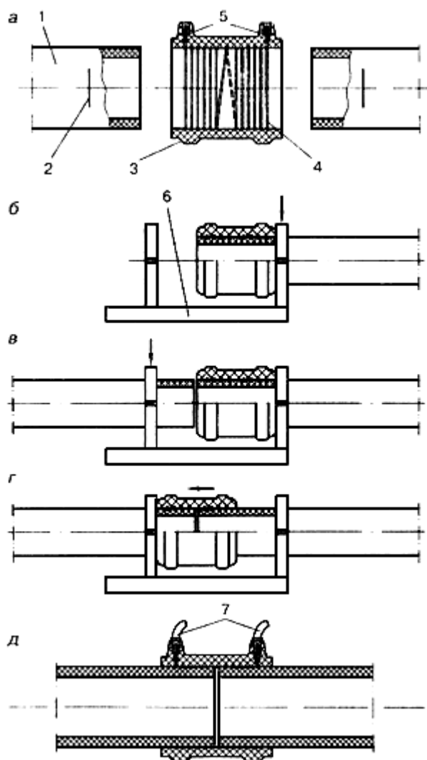
а - подготовка соединяемых элементов; б, в, г - этапы сборки стыка; д - собранный под сварку стык;
