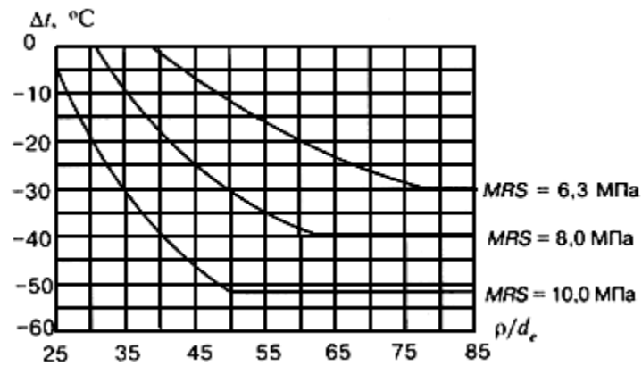
Рисунок 4 - Максимально допустимый отрицательный температурный перепад в зависимости от отношения радиуса упругого изгиба к наружному диаметру газопровода при температуре эксплуатации 0 °C и рабочем давлении 0,3 МПа для SDR 11 и различных MRS
