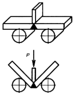
Рисунок Ф.1 - Схема испытания на статический изгиб
